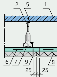
Stoß an den Stirnkanten
