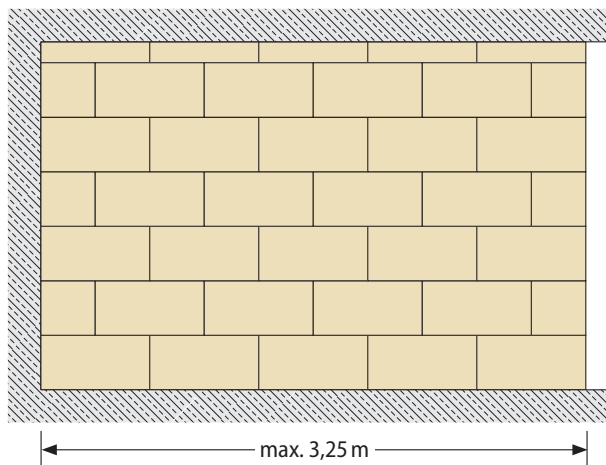
3-seitige Lagerung mit Deckenanschluss
